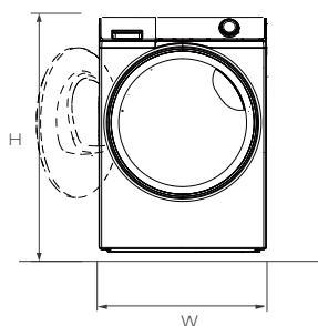
ВИД СПЕРЕДИ
