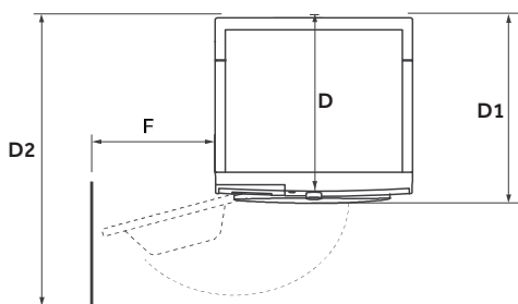
ВИД СВЕРХУ
