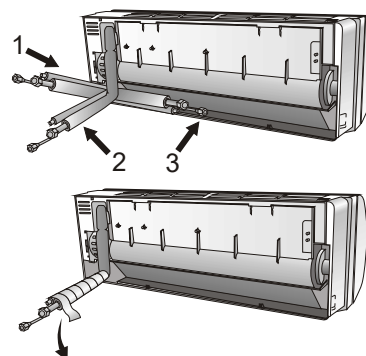
Возможные направления прокладки трубопровода
