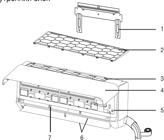
Внутренний блок
