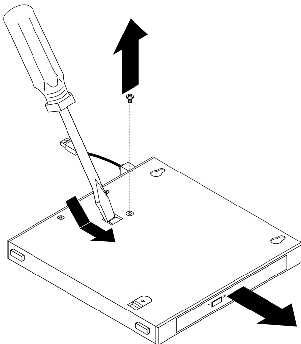
Рис. 18. Извлечение внешнего дисковод для оптических дисков из корпуса
