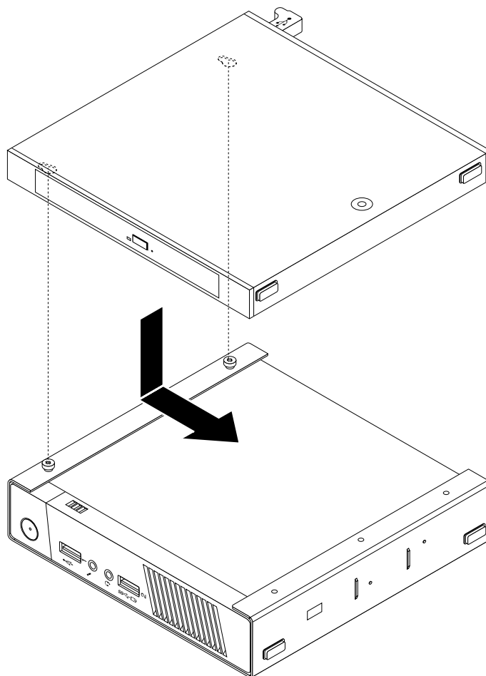
Рис. 33. Установка корпуса дисковод для оптических дисков
