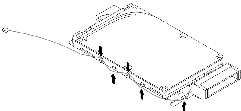
Рис. 61. Прокладка кабеля передней антенны Wi-Fi
