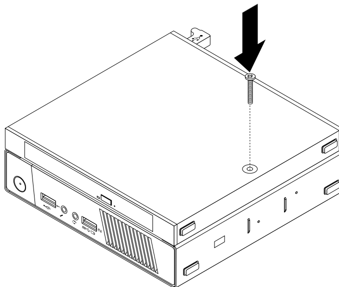
Рис. 24. Установка винта, который фиксирует корпус внешнего дисковод для оптических дисков
