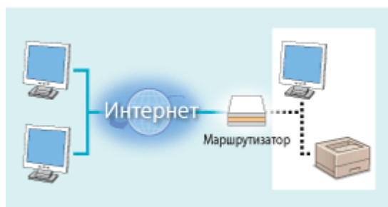
Частный IP-адрес
