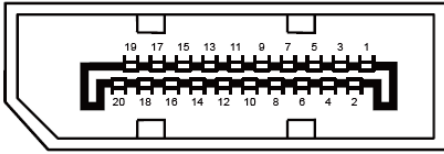
20-контактный кабель для передачи сигналов цветного изображения
