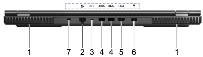
Рис. 8. Вид сзади - 17-дюймовые модели
