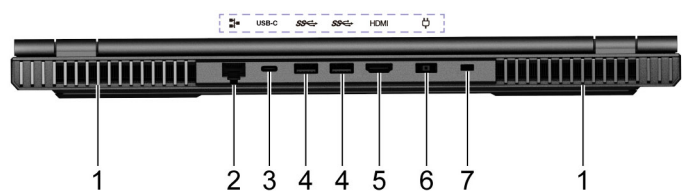
Рис. 7. Вид сзади - 15-дюймовые модели
