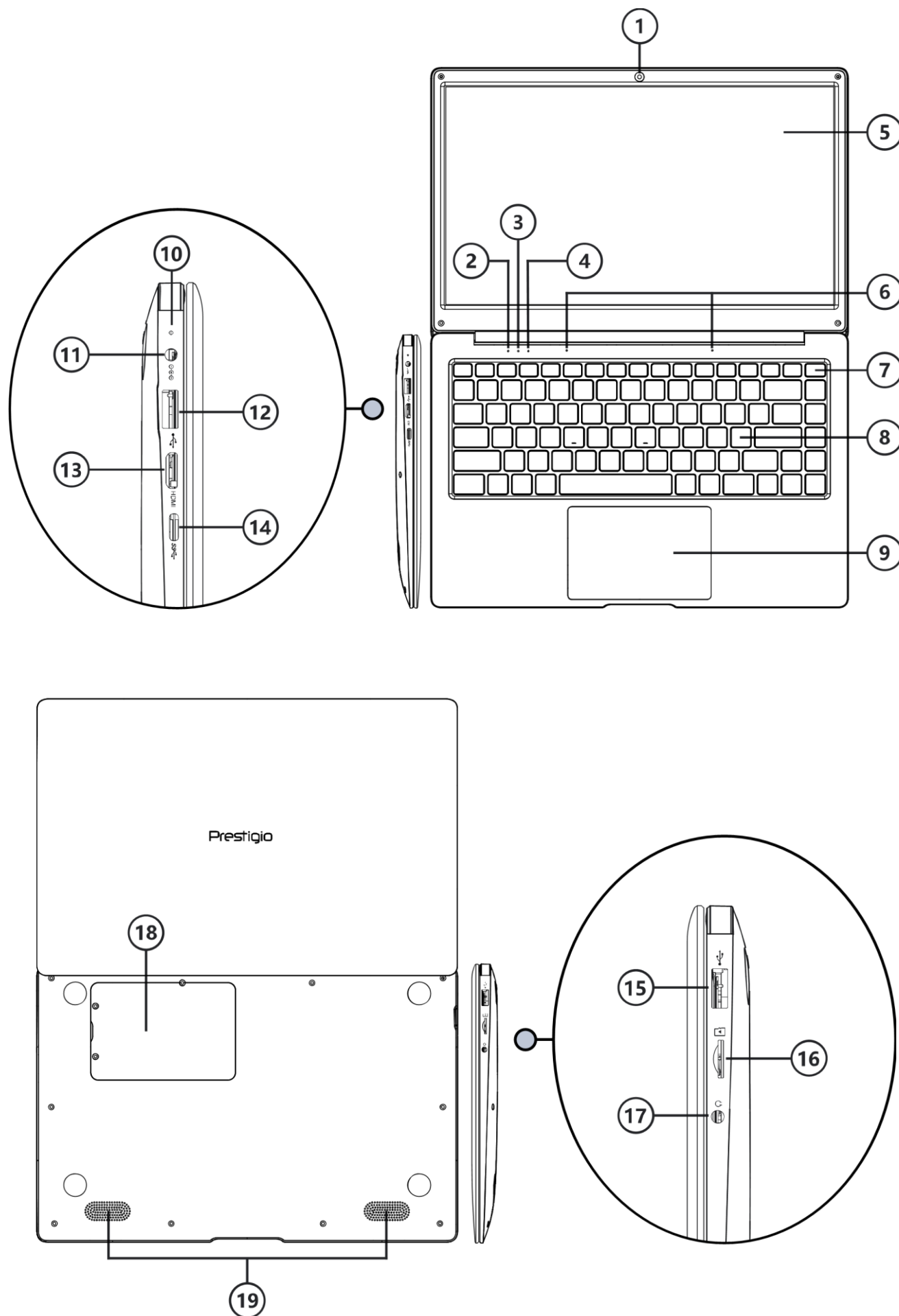
Рисунок 2 – Компоненты и элементы управления
