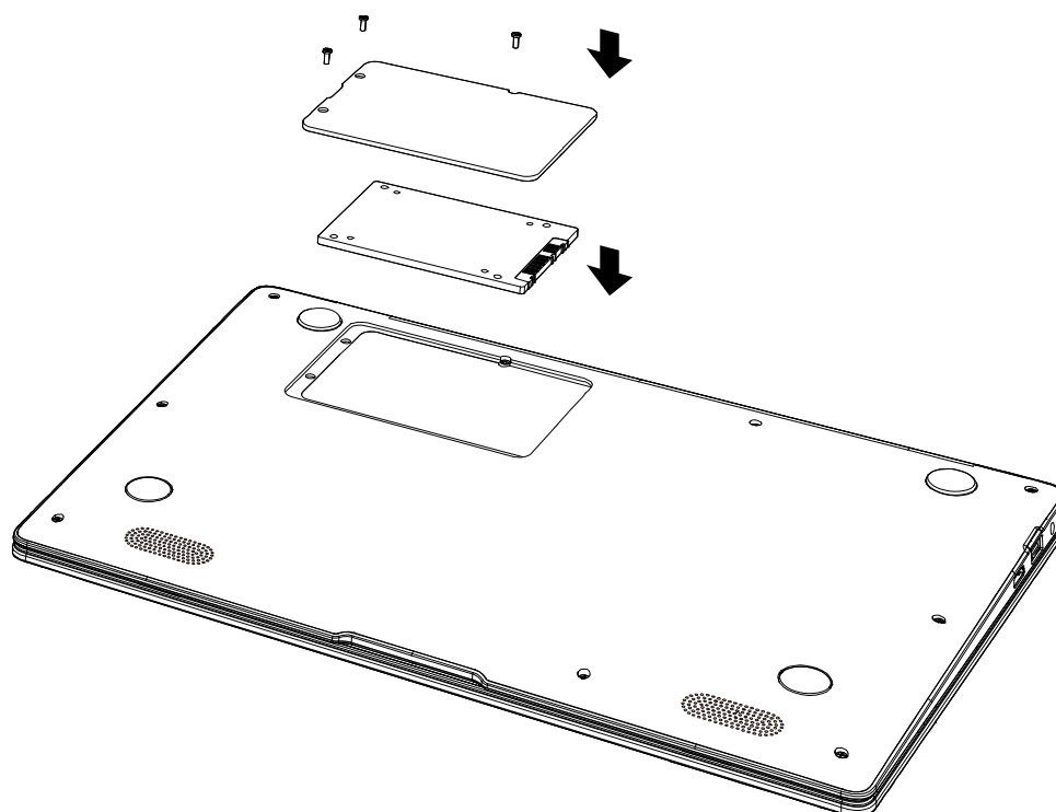
Рисунок 8 – Установка накопителя
