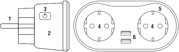
1 – вилка для подключения к сети; 2 – корпус; 3 – кнопка включения/выключения; 4 – розетка для подключения нагрузки; 5 – светодиодный индикатор; 6 – USB-разъемы.
