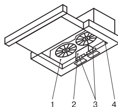
Рис. 2. Kamilla slim 600 ЗР, Kamilla slim 600 (2 мотора)
