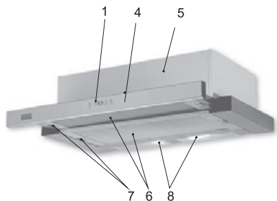
Рис. 1. Kamilla slim 600 ЗР
