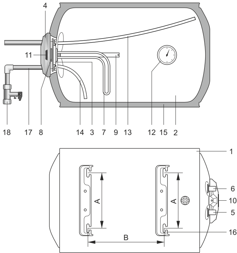
Рис. 2. Горизонтальное размещение
