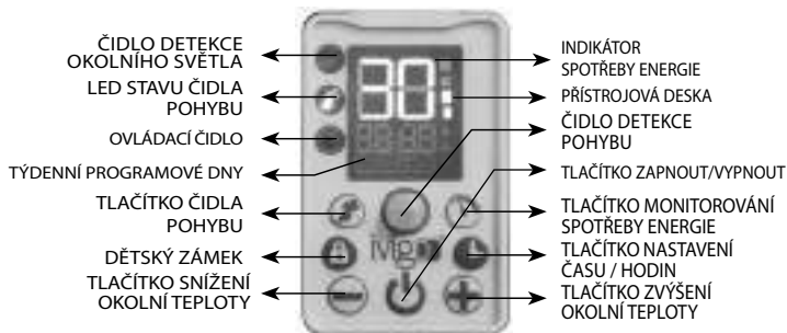
Obrázek 10. Elektronický ovládací panel profesionálního konvektorového topidla
