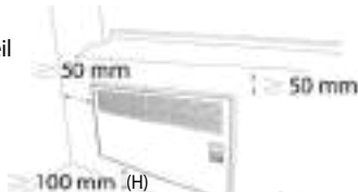
Bild 4. Mindestabstände für eine effiziente Funktionstüchtigkeit des Gerätes
