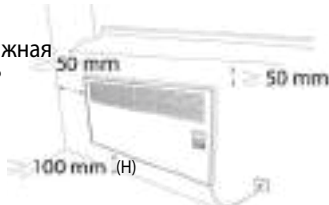
Рисунок 4. Допустимое расстояние
