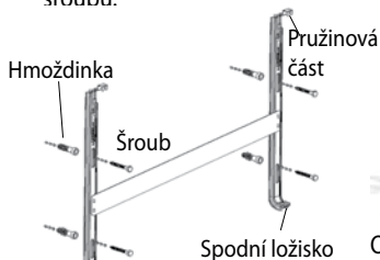
Obrázek 3. Závěsné háky
