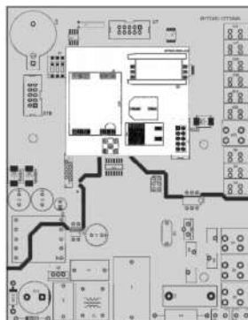
Рис 3. Вид платы с установленным GSM модулем
