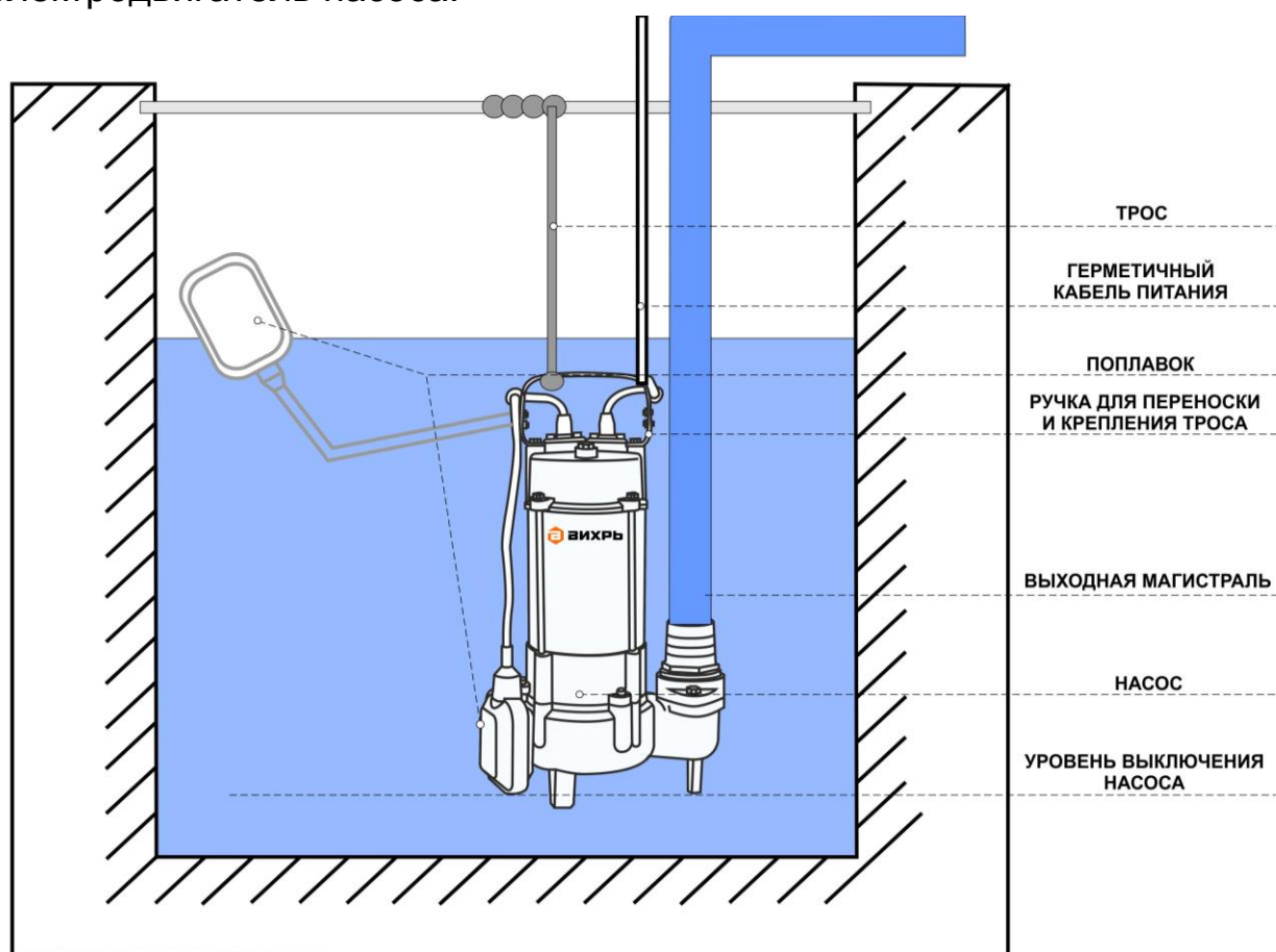
Рис.2 Монтаж насоса
