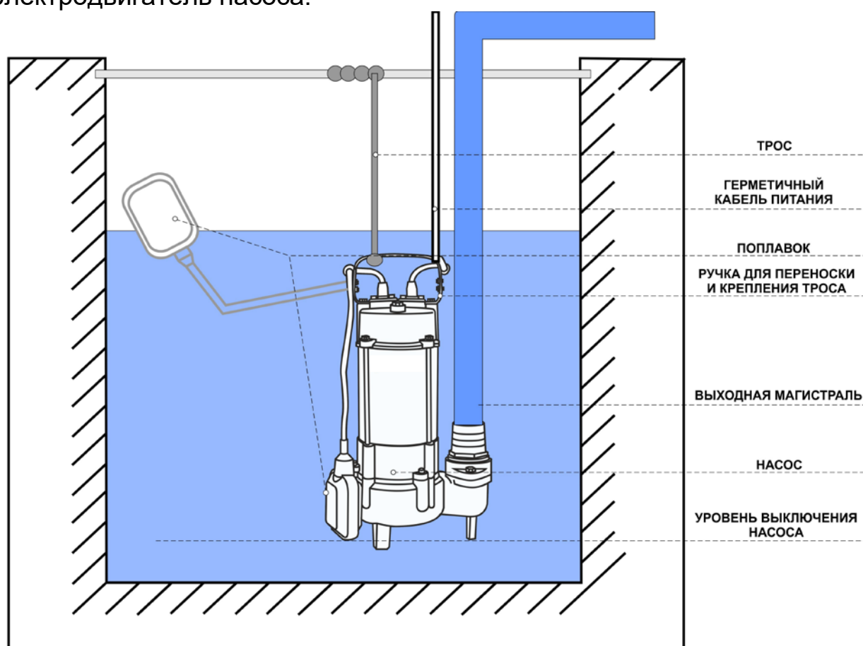
Рис.2 Монтаж насоса
