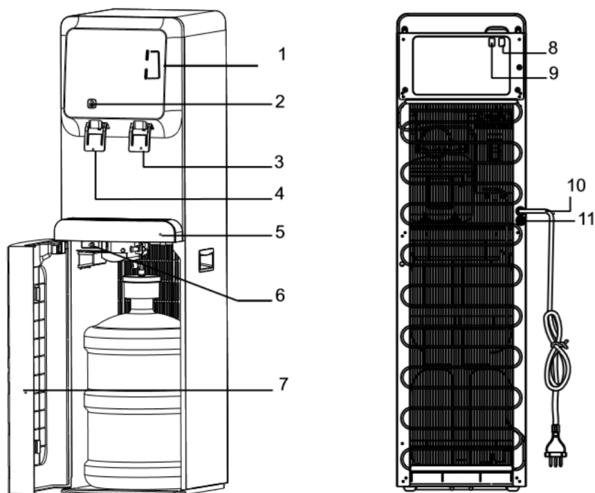
Рис. 1. Схема аппарата V800AE
