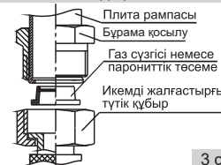
Икемді қосылыс
