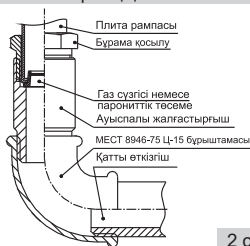
Икемді қосылыс
