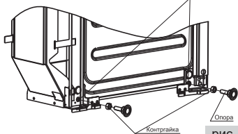
Установка регулируемых опор (вид снизу)
