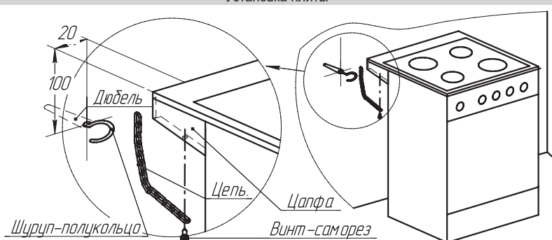
Установка плиты
