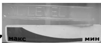
Метка минимального и максимального уровня масла
