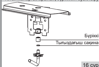
Үстел жанарғыларының бүріккісін ауыстыру
