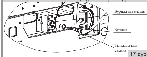
Оттық жанарғысының бүріккісін ауыстыру
