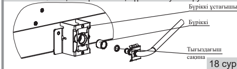
Оттық жанарғысының бүріккісін ауыстыру
