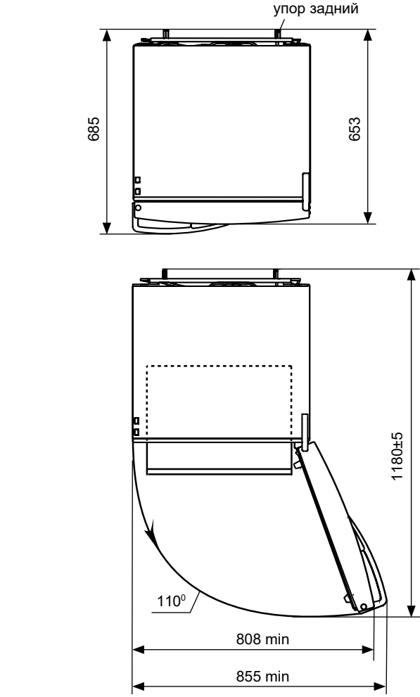
Рисунок 2 – Холодильник (вид сверху)
