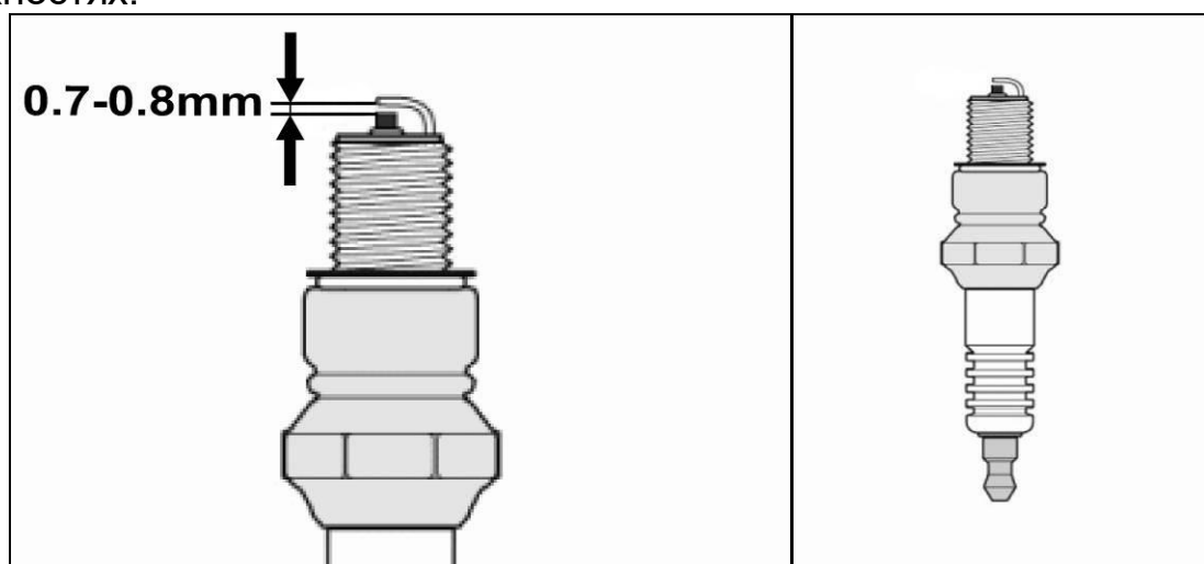
Рис. 29. Свеча зажигания
