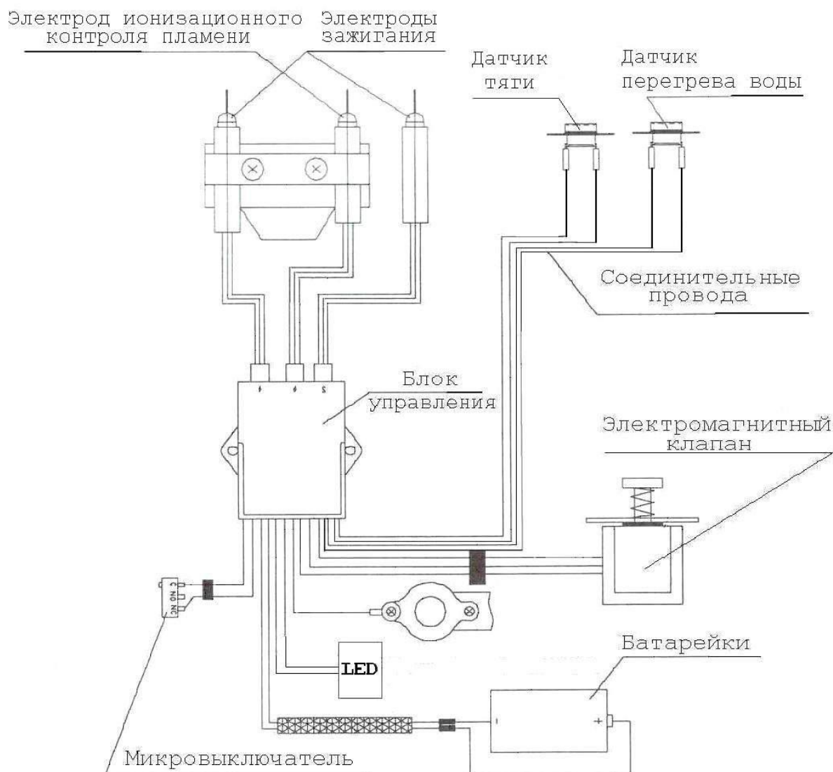
Рис. 2. Схема электрическая
