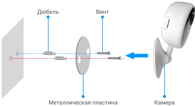
Рисунок 2. Монтаж на шурупы
