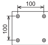
Рисунок 4 – Размеры для выбора настенного кронштейна
