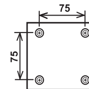
Рисунок 4 – Размеры для выбора настенного кронштейна
