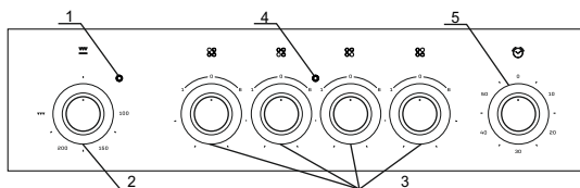
Панель управления плит моделей 506004.13эс-001, 506004.13эс-002
