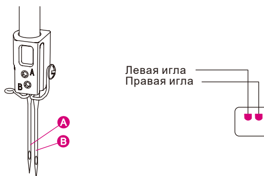
Левая и правая иглы
