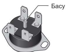
3-сурет. Термоажыратқыш.
