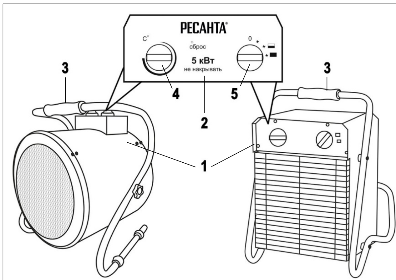
Рис. 1. Общий вид.
