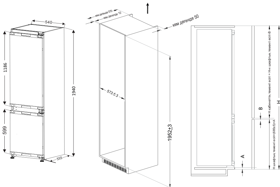
ЖИҢАЗ ФРОНТЫ МЕН ТОҢАЗЫТҚЫШТЫҢ ӨЛШЕМДЕРІ
