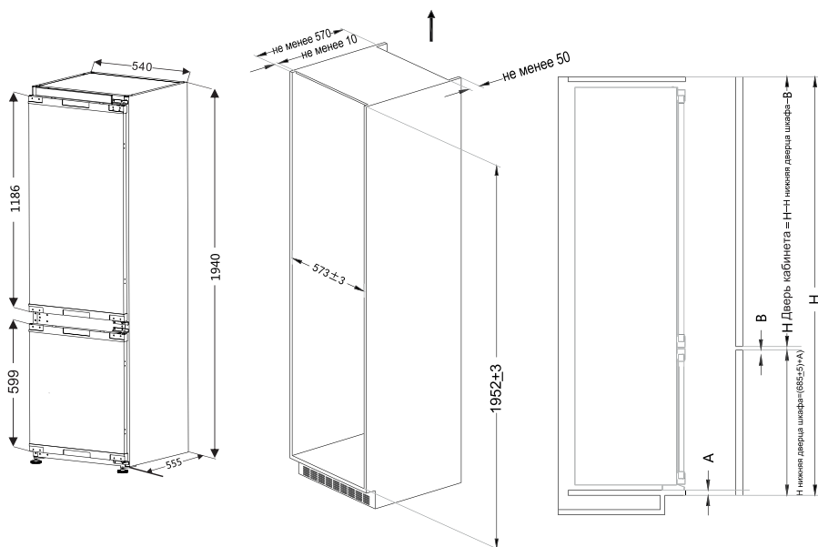
ГАБАРИТЫ МЕБЕЛЬНОГО ФРОНТА И ХОЛОДИЛЬНИКА
