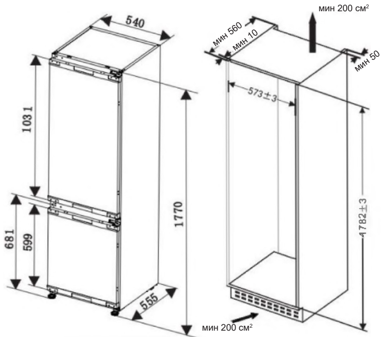
ГАБАРИТЫ МЕБЕЛЬНОГО ФРОНТА И ХОЛОДИЛЬНИКА
