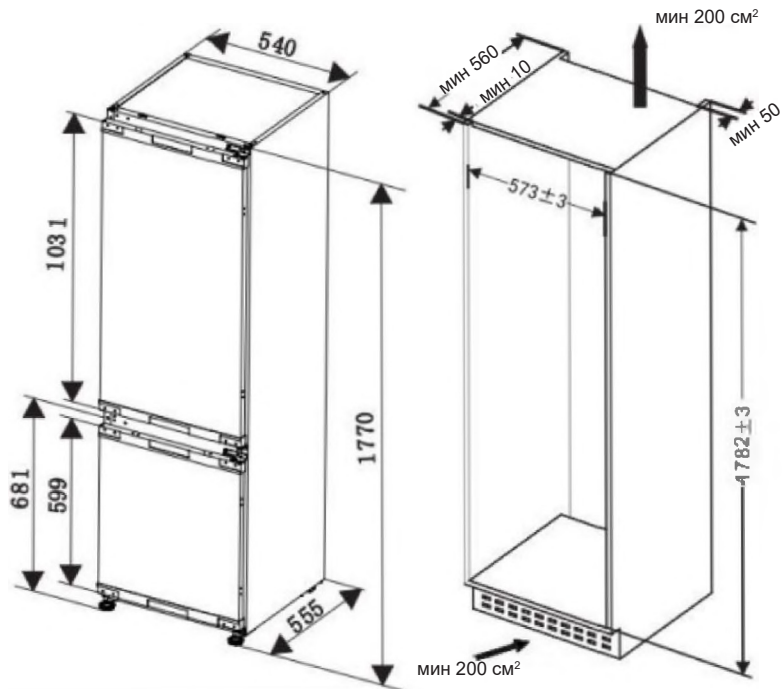
ЖИҢАЗ ФРОНТЫ МЕН ТОҢАЗЫТҚЫШТЫҢ ӨЛШЕМДЕРІ
