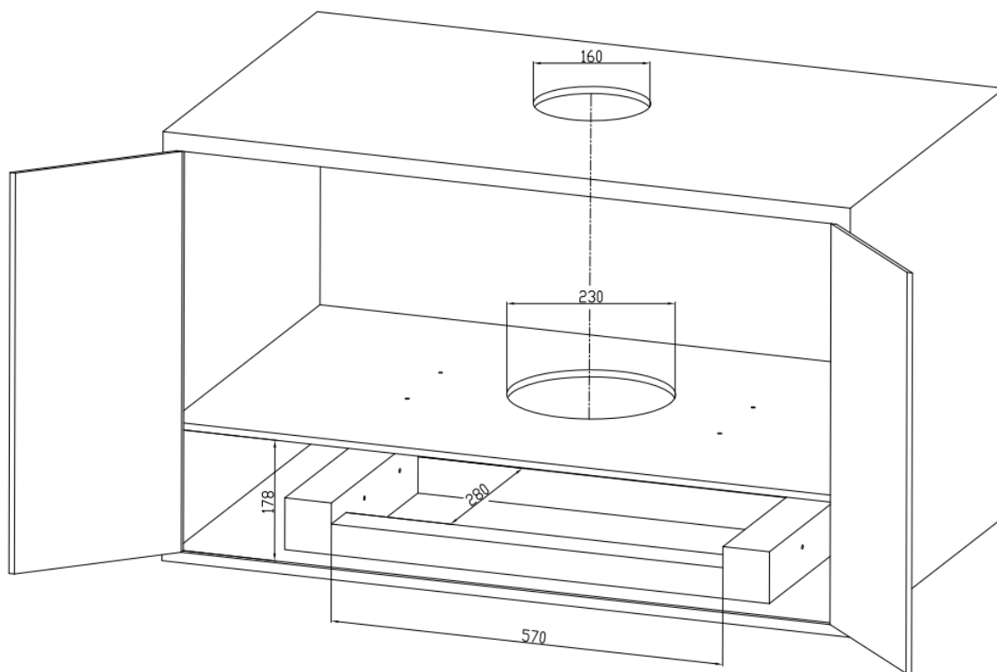
Рис 2. Шкафчик для установки
