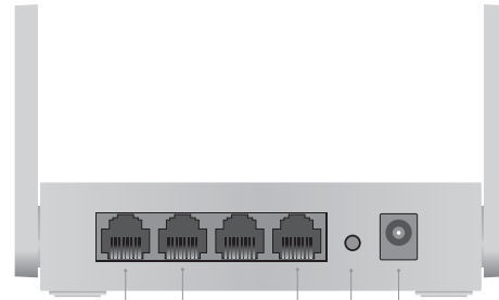
Порт WAN Порты LAN Кнопка WPS Разъём питания
