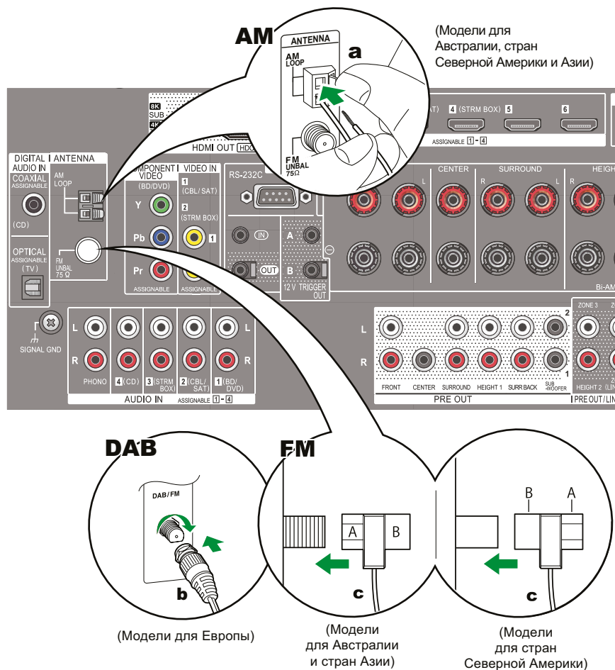
a Рамочная AM-антенна, b DAB/FM-антенна, c Комнатная FM-антенна
