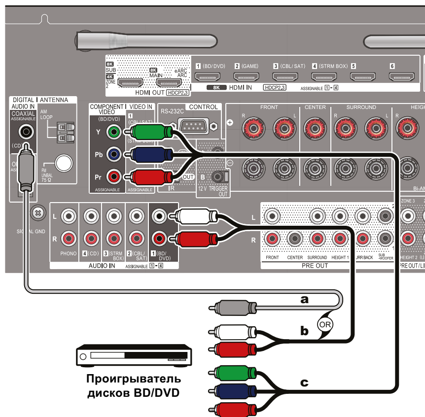
a Цифровой оптический кабель, b Аналоговый аудиоканал, c Компонентный видеоканал
