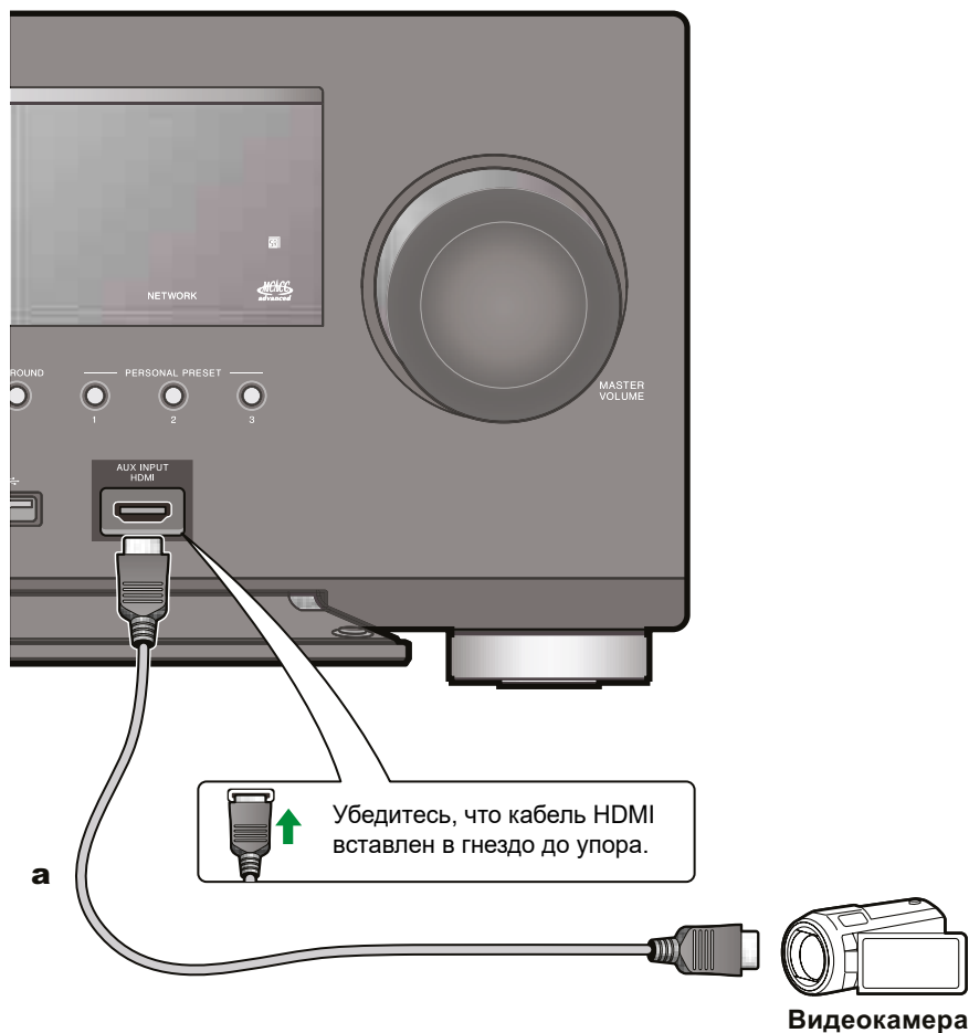
а Кабель HDMI
