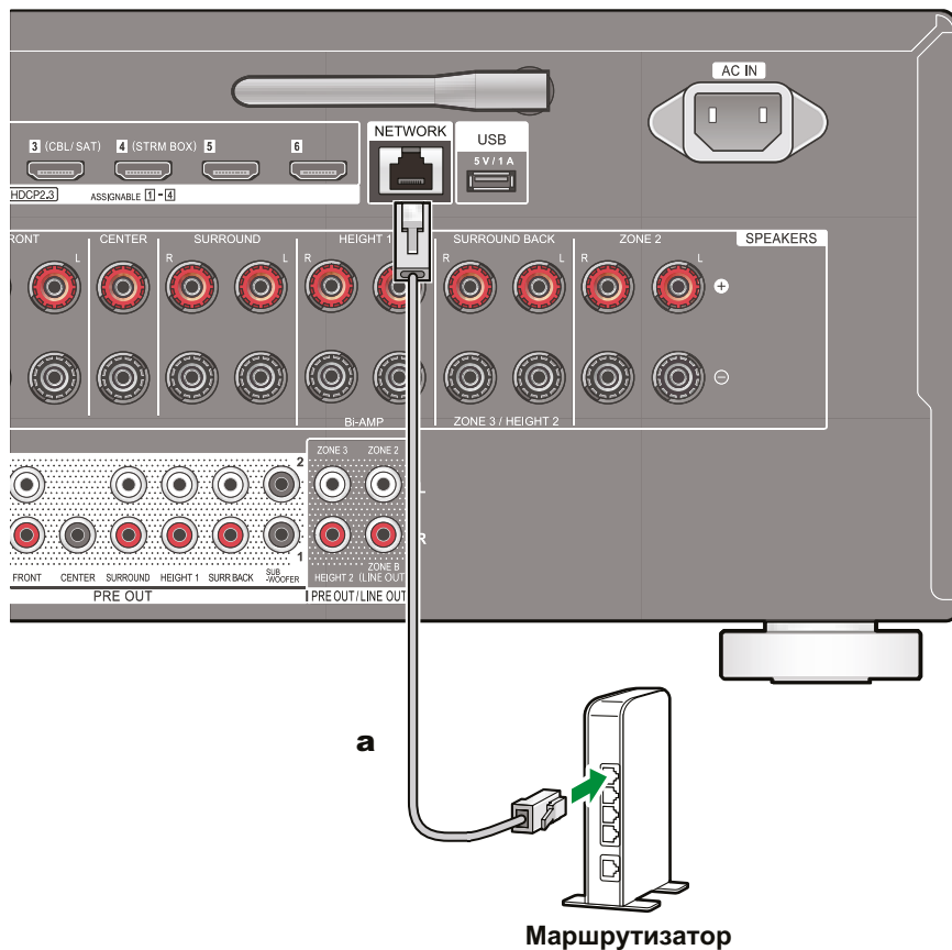
a Ethernet-кабель
