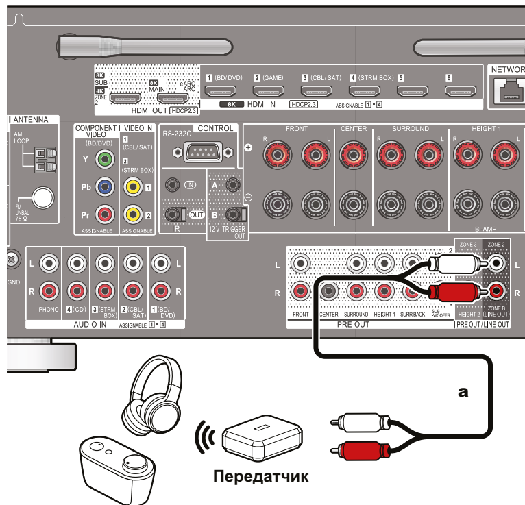
a Аналоговый аудиокабель
