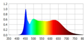
Рис.2 Световые спектры фитосветильника
