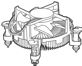
Ветилийтор процессора
