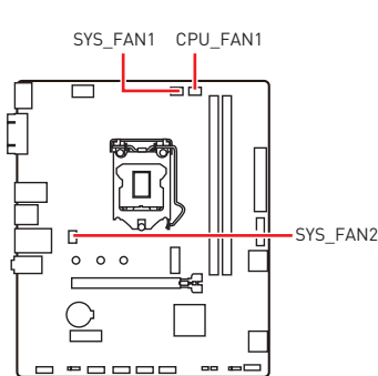
風扇接頭規格
