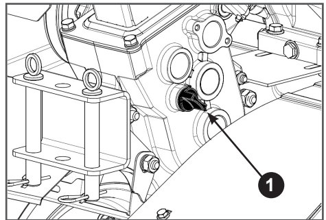
Рис. 25 Крышка маслосливного отверстия редуктора
