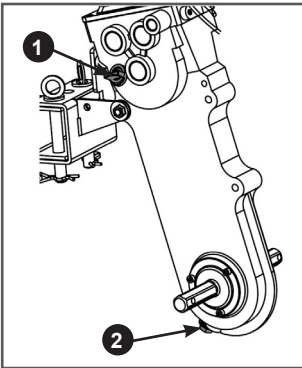
Рис. 39 Замена масла в редукторе
