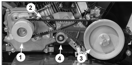
Рис. 40 Замена ремней привода
