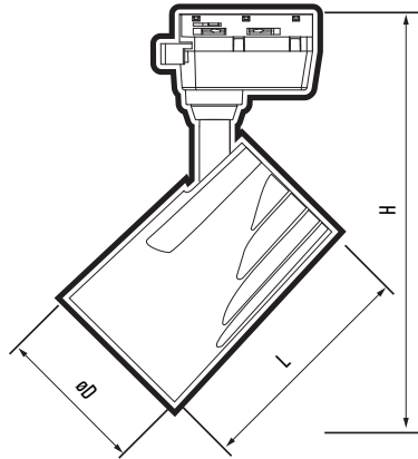
Рис 1. Прожектор PTR 17
