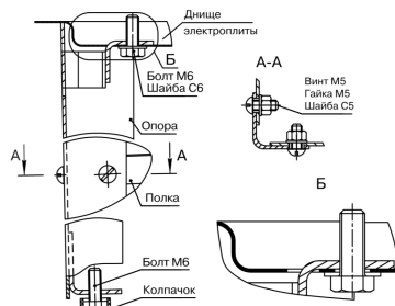
Рисунок 5 — Сборка подставки
