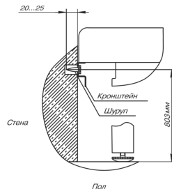
Рисунок 4 — Схема крепления плиты к стене
