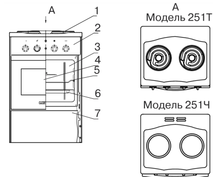
1 — плита с электроконфорками; 2 — панель блока управления; 3 — электрошкаф жарочный; 4 — дверца электрошкафа жарочного; 5 — решетка; 6 — противень; 7 — ящик выдвижной или отсек хозяйственный. Рисунок 3 — Внешний вид плит моделей 251Т, 2514
