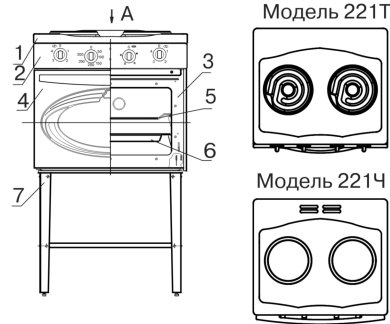
Рисунок 2 — Внешний вид плит моделей 221Т, 221Ч
