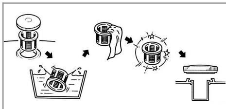
Рис. 18 Обслуживание сетчатого фильтра в горловине топливного бака
