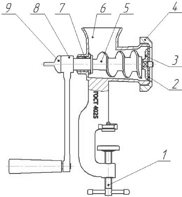
Рисунок 1- Устройство изделия
