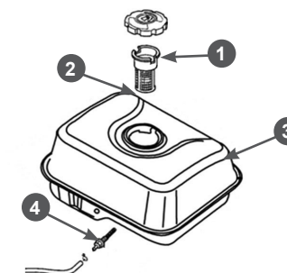
Рис. 14 Топливные фильтры
