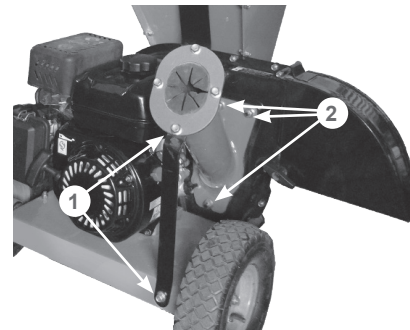
Рис. 20 Снятие воронки измельчителя
