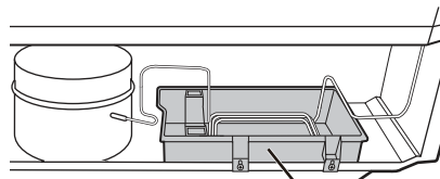
Испарительный лоток
