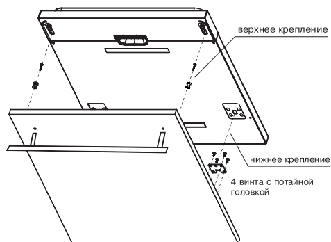
Рис. 3а. Установка декоративной панели.
