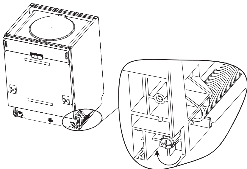
Рис. 4. Регулировка натяжения пружины дверцы
