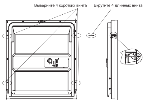
Рис. 3б. Крепление декоративной деревянной панели.
