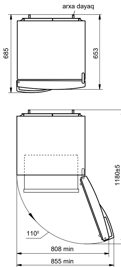
Şəkil 2 – Soyuducu (üstən görünüşü)
