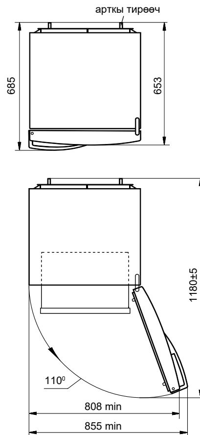
2-сүрөт – Муздаткыч (үстүнөн көрүнүшү)
