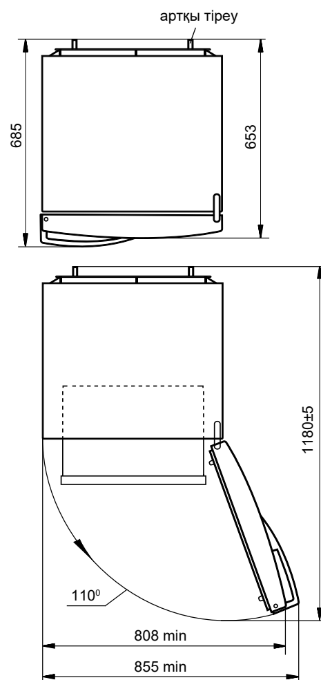
2-сурет – Тоңазытқыш (жоғарыдан қарау)
