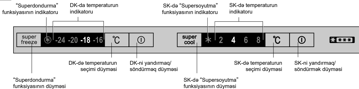
Şəkil 3 – İdarəetmə paneli
