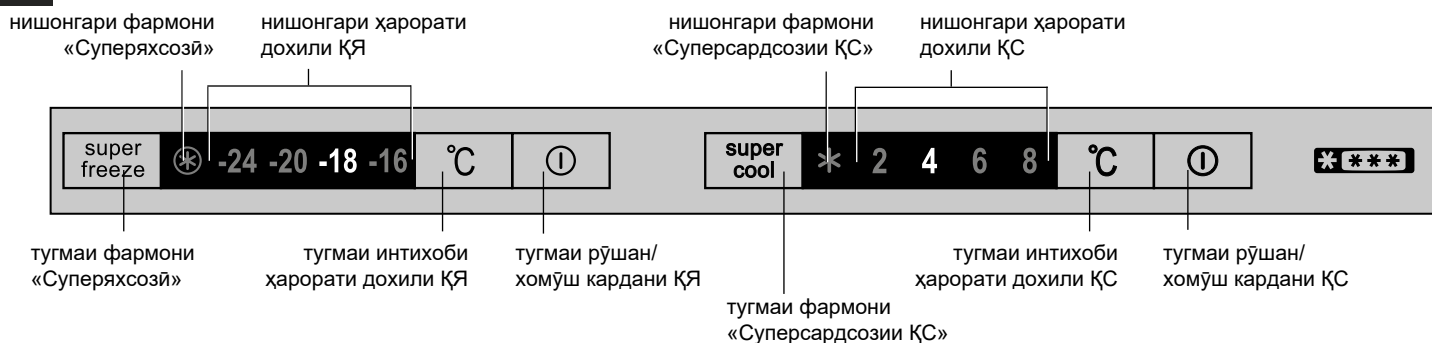
Тасвири 3 – Тахтаи фармонҳо
