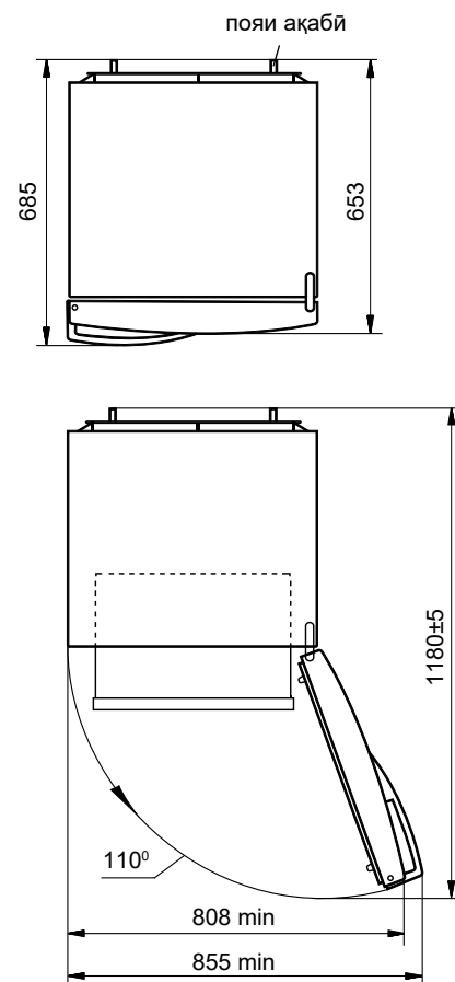
Тасвири 2 – Яхчол (намо аз боло)
