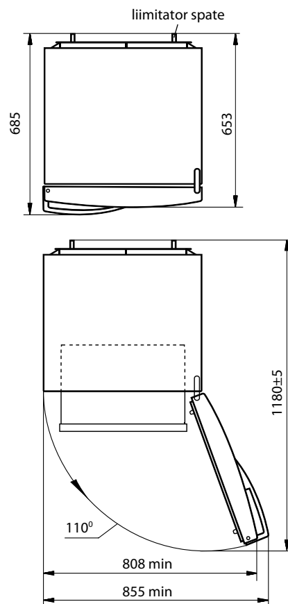
Figura 2 – Frigider (vedere de sus)
