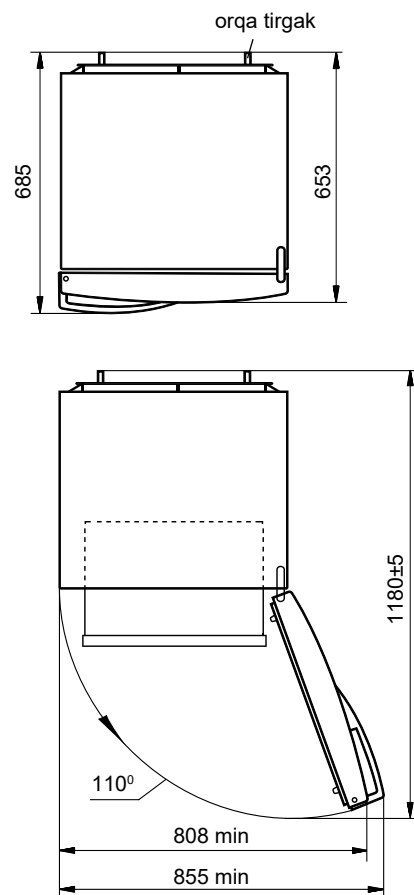
2-rasm – Sovutgich (yuqoridan ko'rinish)
