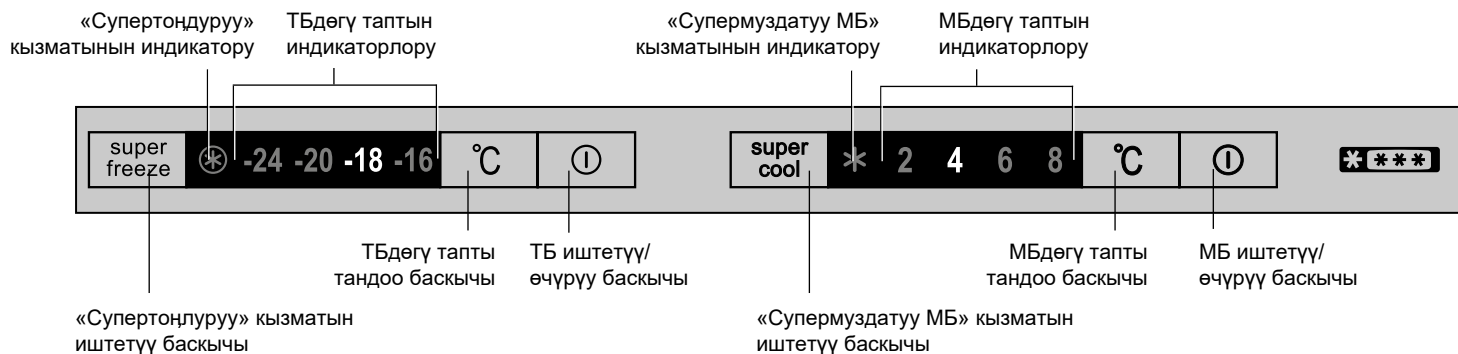
3-сүрөт – Башкаруу панели
