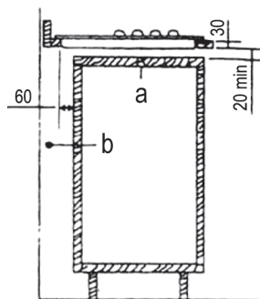
a – жылжымалы панель b – қосылуға арналған кеңістік
