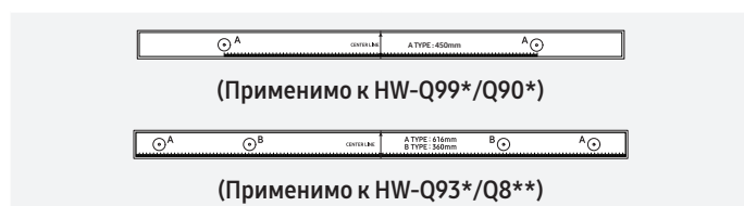
Ⓐ Направляющая для настенного монтажа
