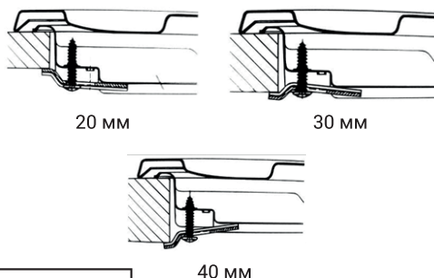
Положение крепежной пластины при разной толщине столешницы
