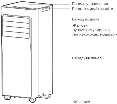
Вид спереди
