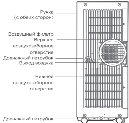
Вид сзади
